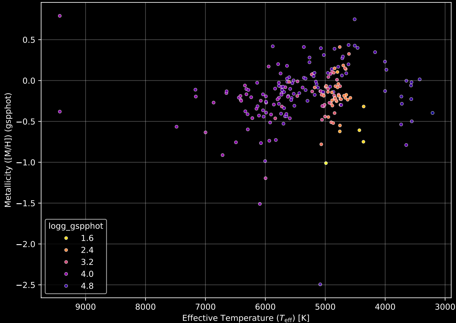
APOGEE DR17 Field: [CVZTILE_092+39_btx] Stellar Population Parameters (n= 204)
